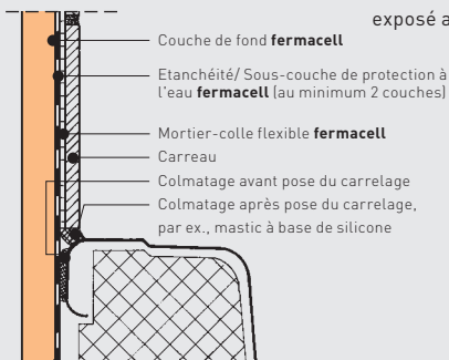
Raccords entre la cabine de douche ou la baignoire et le mur Raccord avec panneau de support fermacell simple
