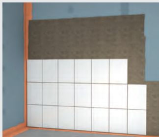
Fig. 22 : Utilisation de Plaques fermacell Powerpanel H 2 O en intérieur. Les carreaux sont posés sur une fine couche de Mortier-colle flexible fermacell (protégeant contre une taux d'humidité de classe A01).
