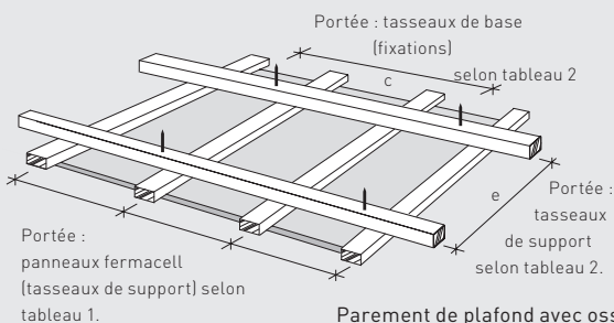
Faux-plafond avec ossature métallique, suspendu
