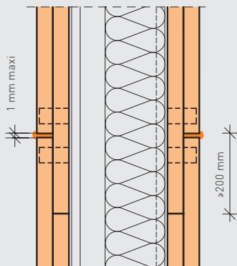
1 o couche/couche intérieure fixée sans colle 2 e couche/couche extérieure collée
