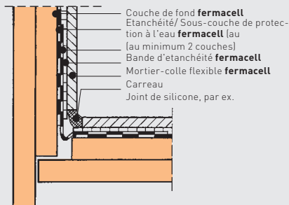
Raccord d'angle exposé aux projections
